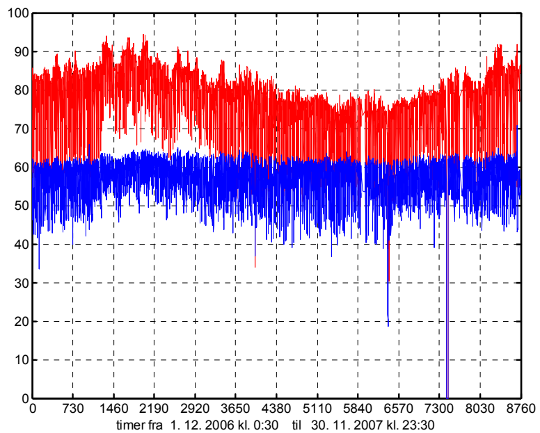
Figur B.2.21.7. Fjernvarmetemperaturer til varmtvandskredsen (før anlægshunt) (timeværdier)
