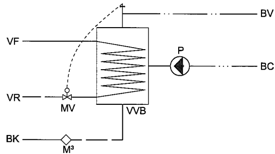
Figur 2.2.4. Varmtvandsproduktion, beholderløsning.
