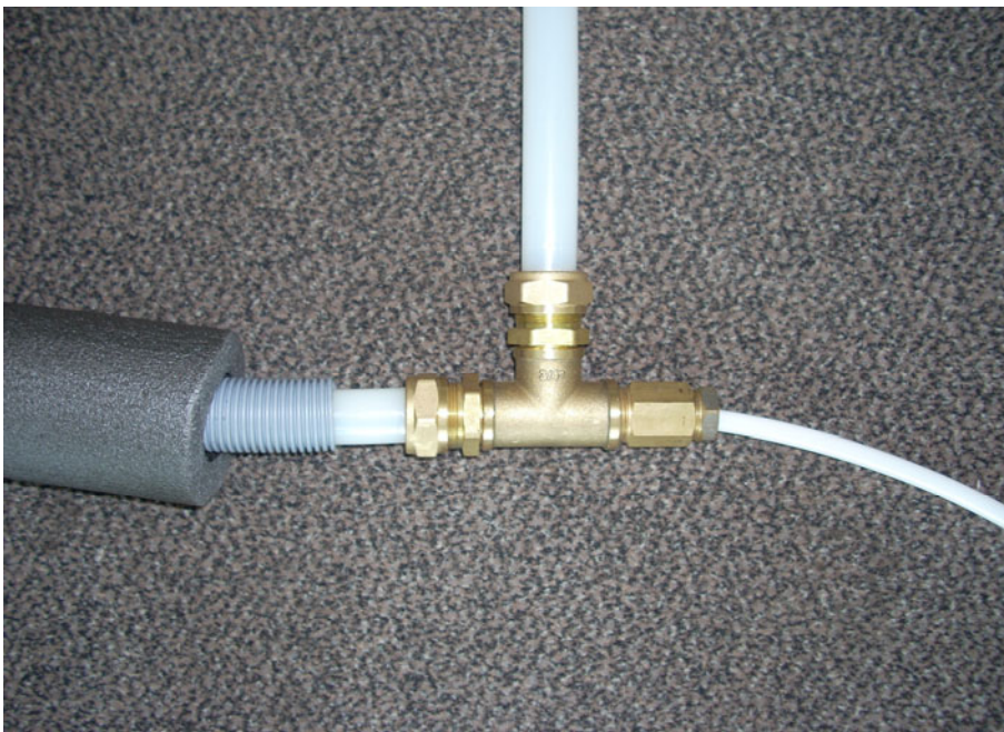
Figur 2.4.6. Rør-i-rør, pex-pex (Foto: Golan Plastic Products).
