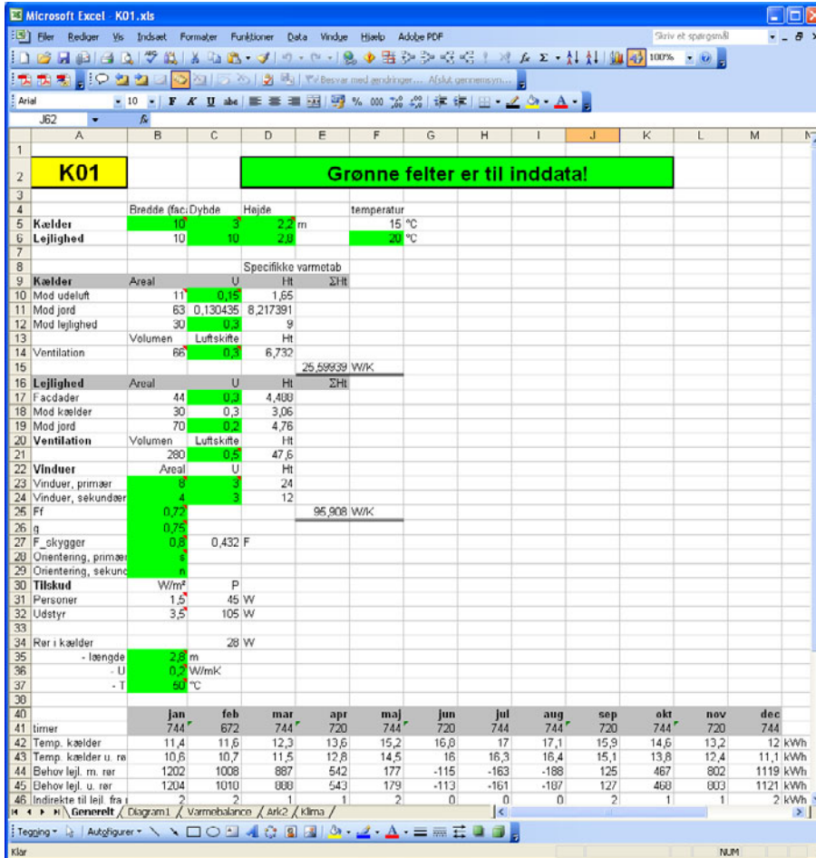
Figur B.4.2.2. Skærbillede fra beregningsmodellen for placering af rør til varmt vand gennem en kælder under et beboelsesrum.
