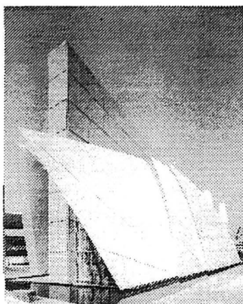
Figur 6. Den Danske Pavillon i Sevilla og randværdien for en simplificeret model.
