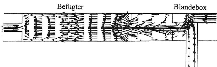
Figur 12. Strømningssimulering af blandebox og befugter, Alamdari [20].
