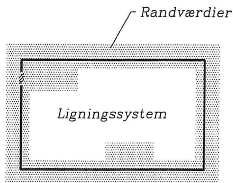
Figur 4. Randværdier omkring et løsningsfelt for strømningsberegning.
