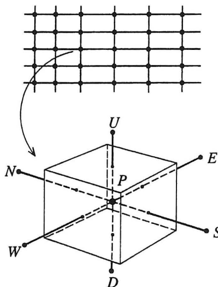
Figur 2. Netpunktsfordeling samt kontrolvolumen omkring et enkelt netpunkt P .
