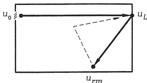
Figur 5. Skitsen illustrerer, hvorledes strømmingen i et givet område hovedsageligt er påvirket af forhold i modstrømsretning, medens den kun er lidt påvirket af det videre forløb via den recirkulerende luftbevægelse.
