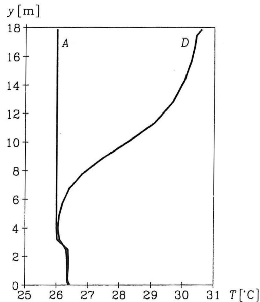
Figur 7. Beregnet lodret temperaturfordeling i udstillingslokale.
