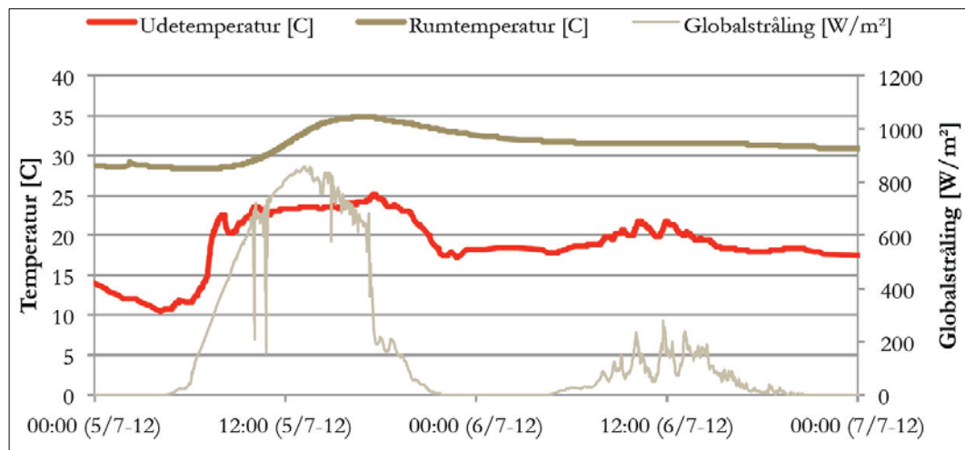
Figur 16. Ude og inde temperatur samt globalstråling for de to forsøgsgdage.
