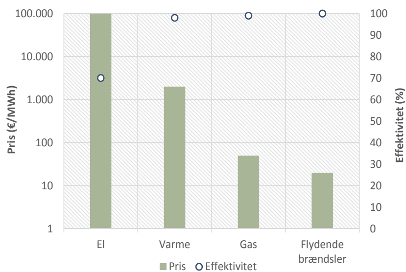
Figur 2. Investeringsomkostninger og effektivitet sammenlignet for forskellige energilagrings teknologier
