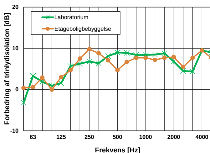
Figur 38. Sammenligning af forbedring af trinlydisolation opnået i laboratorium og i etageboligbebyggelse ved at anvende et underlag af gummimateriale under plastkiler. I begge tilfælde opnås en forbedring på 5 dB på enkelttsværdierne.
