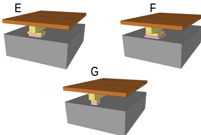
Figur 26. Prøveemner strøgulve med traditionel blød opklodsning, gulv B, og med trinlyddæmpende underlag under opklodsning (Gulve E, F og G).
