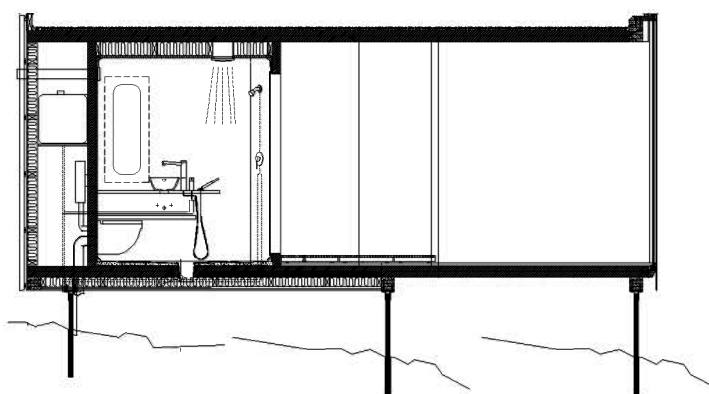
Snitt hytte, Juvet landskapshotell
