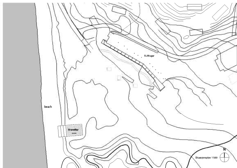
Situasjonsplan.
