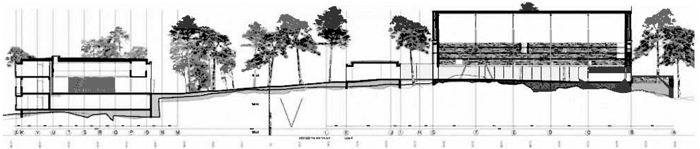
Lengdesnitt, Mortensrud kirke
