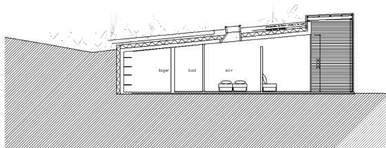
Tverrsnitt.
