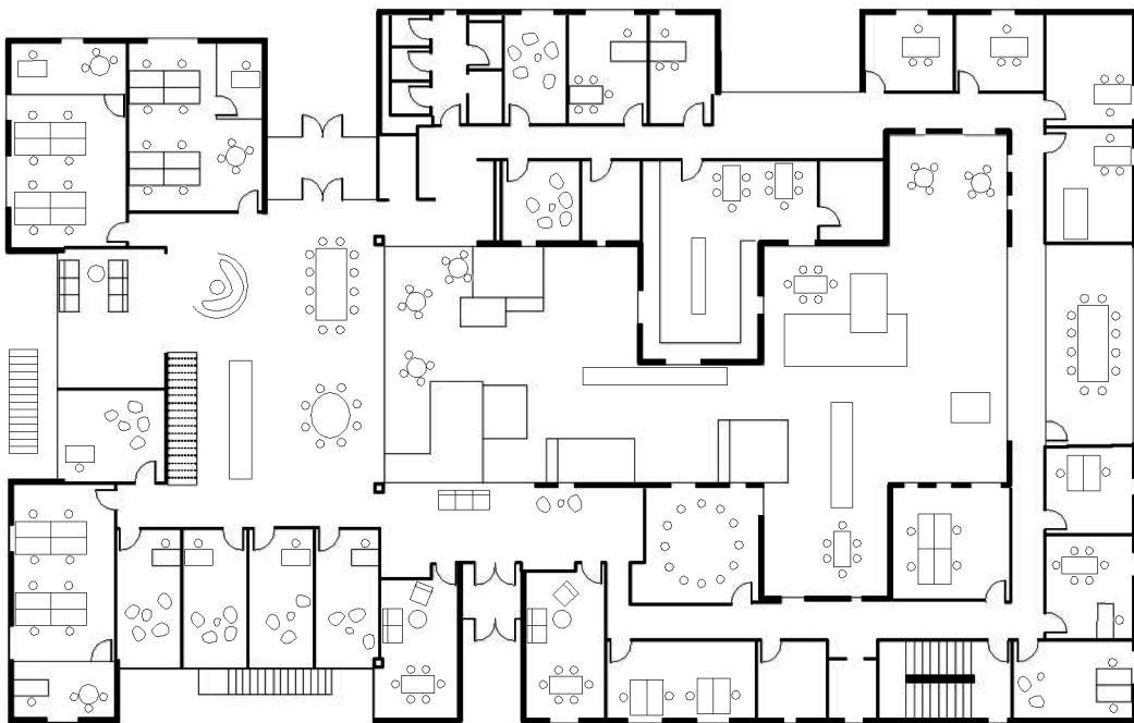
Plan bakkenivå
