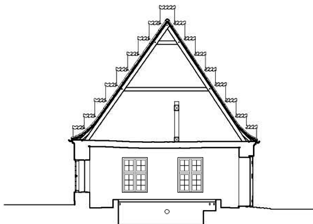
Snitt, bassenget.
