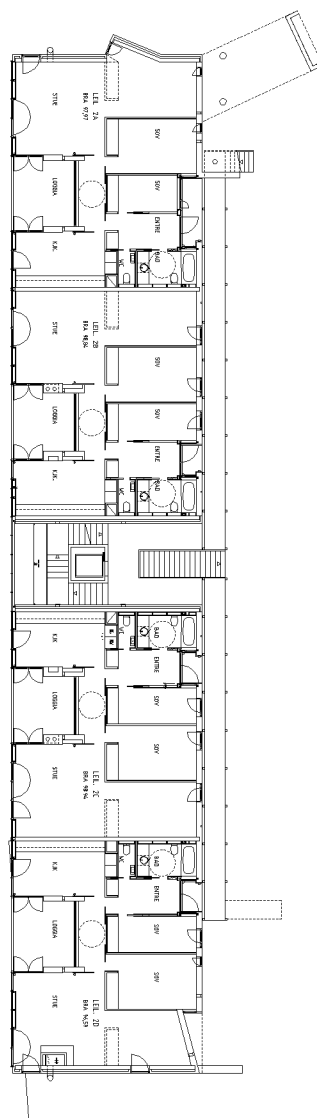
Plan, Bekkelaget 9 B.
