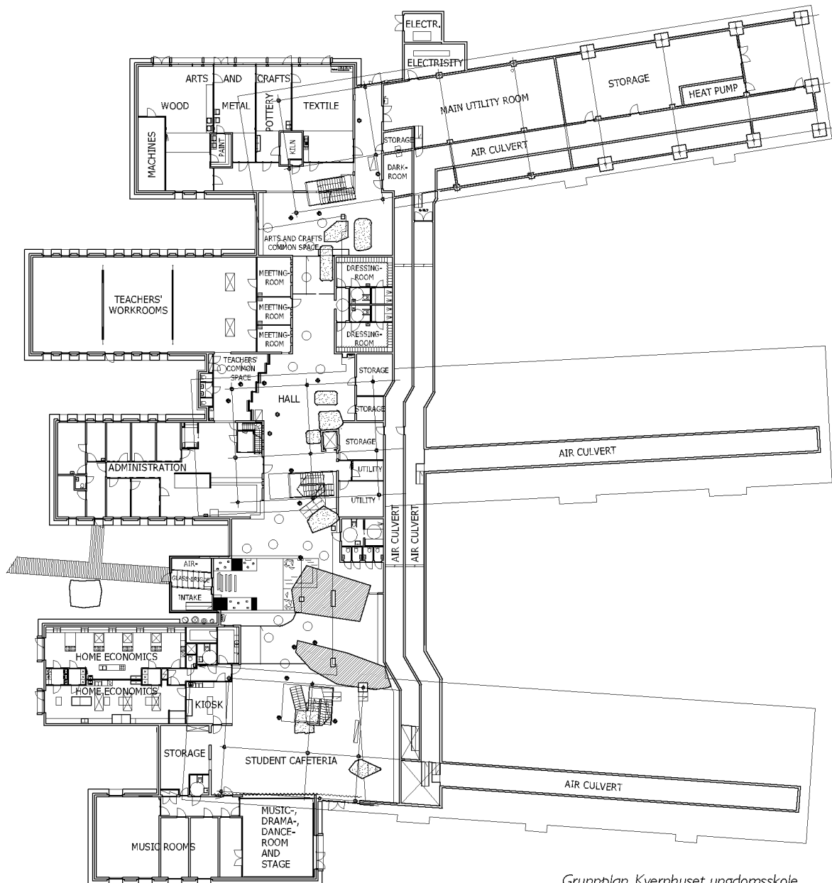
Grunnplan, Kvernhuset ungdomsskole.
