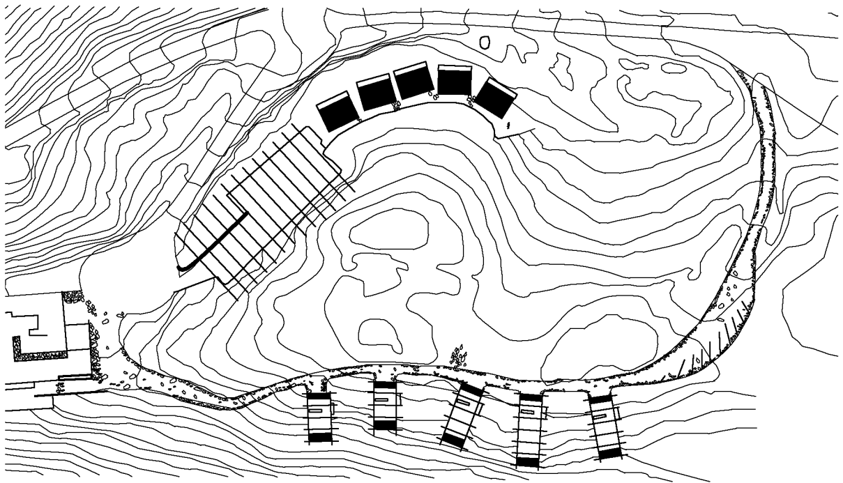
Situasjonsplan, Nordisk kunstsenter.
