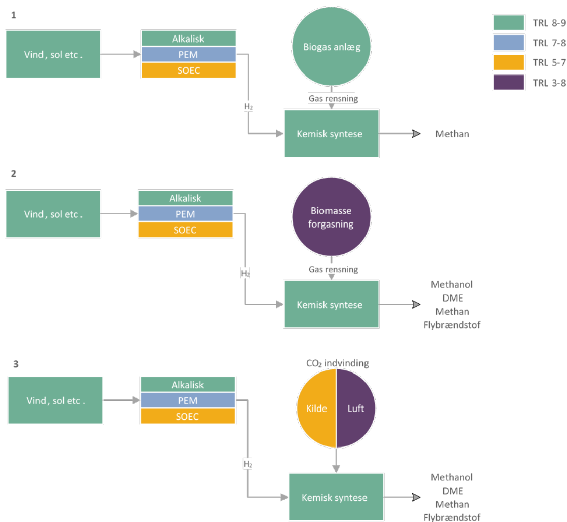
Figur 3. El-til-brændsel konverteringsprocesser med vejledende teknologisk parathedsniveau (forkortet: TRL): 1) biogasopgradering med elektrolyse, 2) biomasse-hydrogenering og 3) CO 2 -hydrogenering til det ønskede brændselsprodukt
