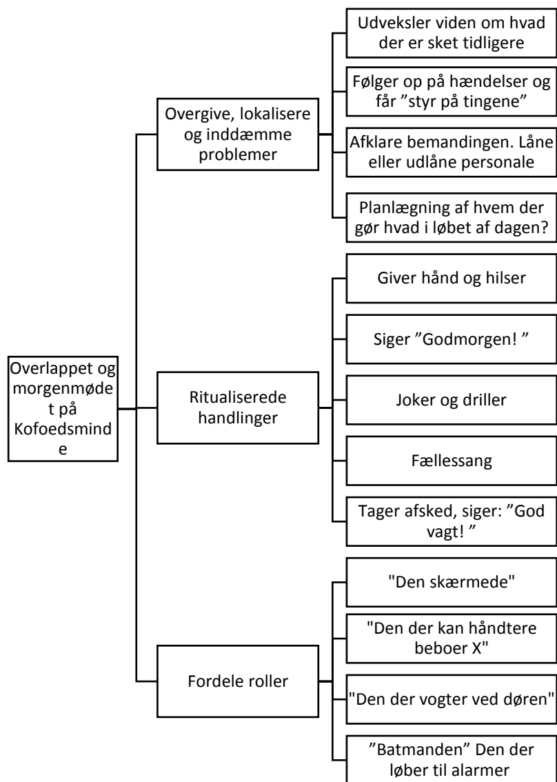
Figur 7 Taksonomi
