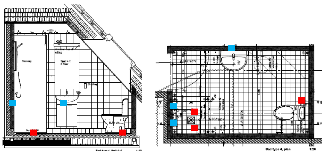
Figur 10. Placering af sensorer i taglejlighed. De blå firkanter markerer placering i vægge og de røde i gulv svarende til tabel 1.
