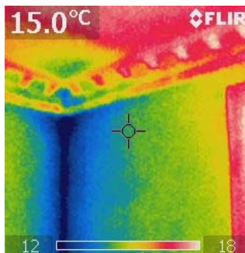
Figur 36. Overgang mellem lejlighedsskel, facade mod gade (til højre) og gavl (til venstre). Det vandrette lejlighedsskel er et traditionelt opbygget træbjækelag med indskud og pudset loft. På det termografiske billede til højre repræsenterer farven rød 18 °C og farven mørkeblå 12 °C. Til venstre er vist et sædvanligt fotografi taget fra samme sted.
