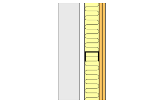
Ny fritstående forsatsvæg. Vandret snit. Skeletkonstruktion / stolper fastgjort på gulv og loft. Tykkelse min. 105 mm. Note: Til murede vægge kan evt. anvendes en forsatsbeklædning, tykkelse min. 80 mm.
