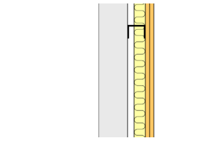
Ny forsatsbeklædning, kun til tunge vægge. Vandret snit. Skeletkonstruktion / stolper på eksisterende væg. Tykkelse min. 80 mm.
