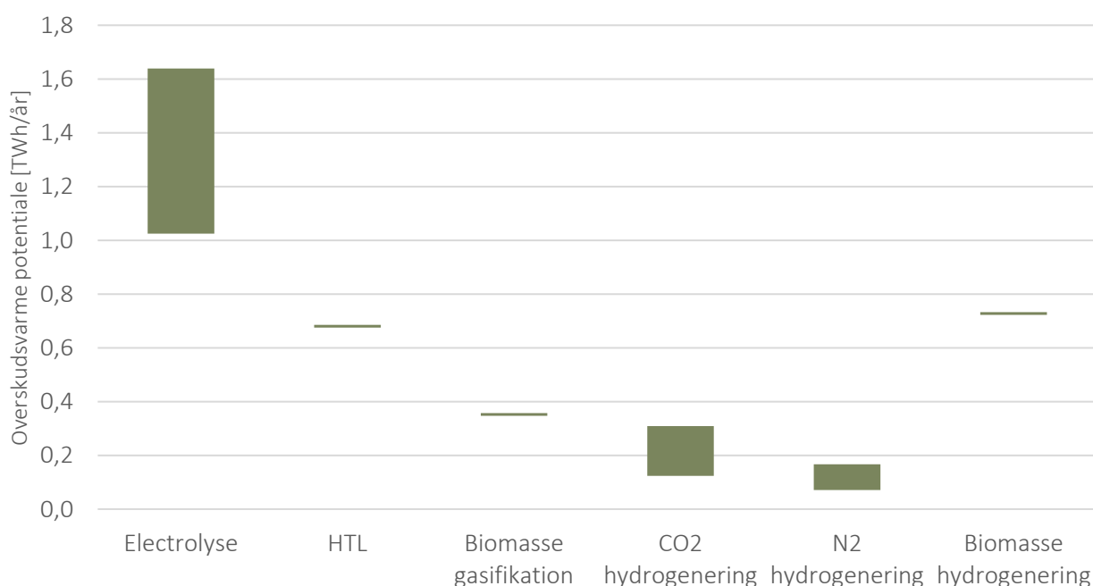
Figur 32: Overskudsvarme potentiale opdelt på Power2X teknologi i IDA 2045.
