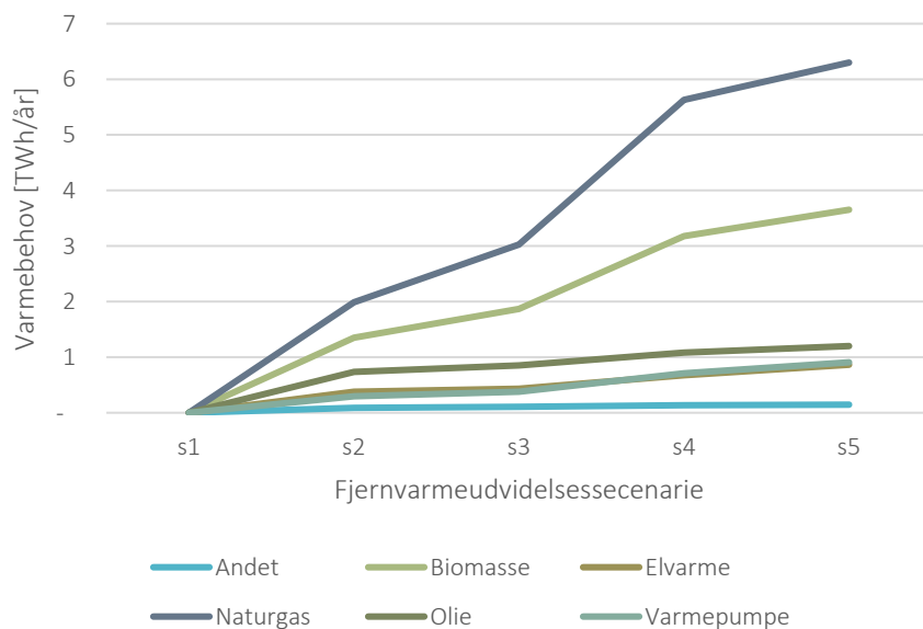
Figur 10: Varmebehov der konverterer til fjernvarme fordelt på forsyningstype og fjernvarmeudvidelsesscenarie, hvis individuel forsynings beholder nuværende forsyning
