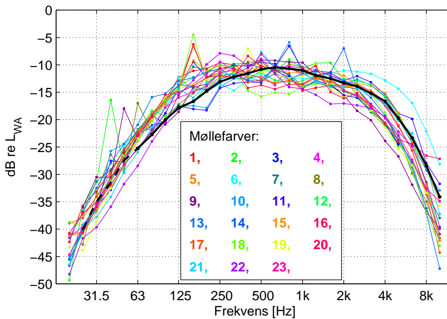
Figur 5. Normerede A-vægtede lydeffektniveauer i 1/3-oktavnband. Gennemsnit af 39 møller \leq 2 MW (tyk sort linje) og 23 individuelle møller > 2 MW.
