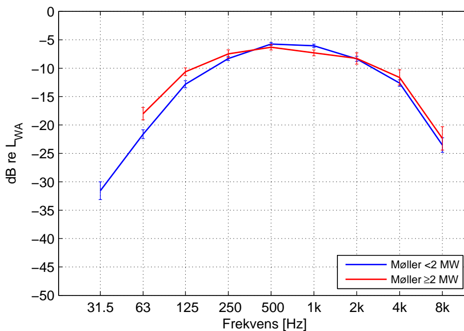
Figur 14. Normeret A-vægtet lydeffektniveau i oktavnåb, gennemsnit for to grupper af møller: < 2 MW og \geq 2 MW. Data fra van den Berg et al. [75, Appendix D]. Lodrette streger viser \pm 1 standard error of mean. (Ingen af de store møller er målt i 31,5-Hz oktavnåb).
