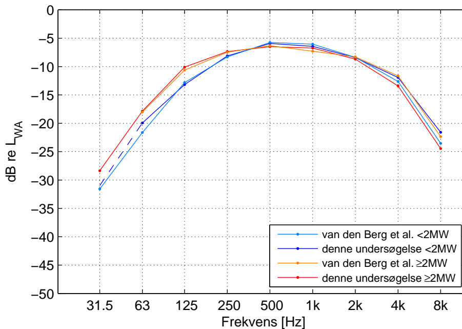
Figur 15. Normeret A-vægtet lydeffektniveau i oktavnåb, gennemsnit for to grupper af møller: < 2 MW og \geq 2 MW og fra to undersøgelser: van den Berg et al. [75, Appendix D] og denne undersøgelse.
