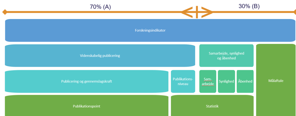
Figur 1 - AAU Forskningsindikator
