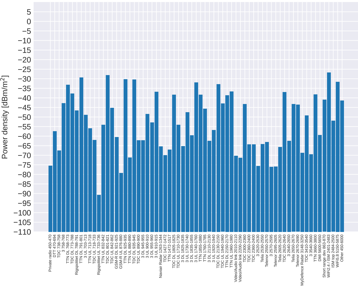
Salling Øverste: Power density
