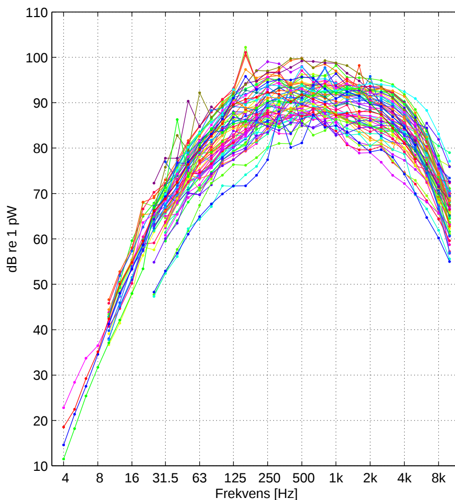
Figur 2. A-vægtede lydeffektniveauer i 1/3-oktavgbånd. 62 møller med nominel elektrisk effekt mellem 75 kW og 3,6 MW.
