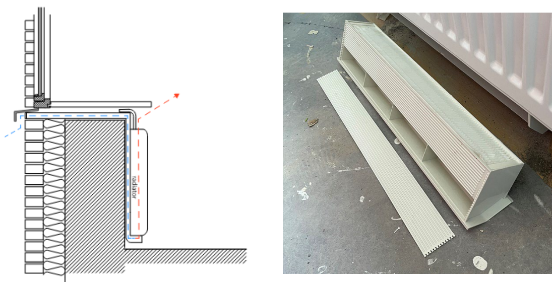
Figur 6. Eksempel på indtag gennem sålbænk i facade med forvarmning gennem radiator samt gennem filterkasse i bund af radiator, snittegning t.v. og foto af filterkasse t.h. Tegning: Purmo. Foto: Mads Gudmand-Høyer.
