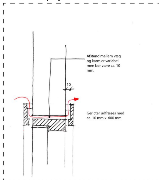
Figur 10. Eksempel på luftoverførsel mellem rum via ventilationsspalte over dørkarm. Tegning: NOVA5.
