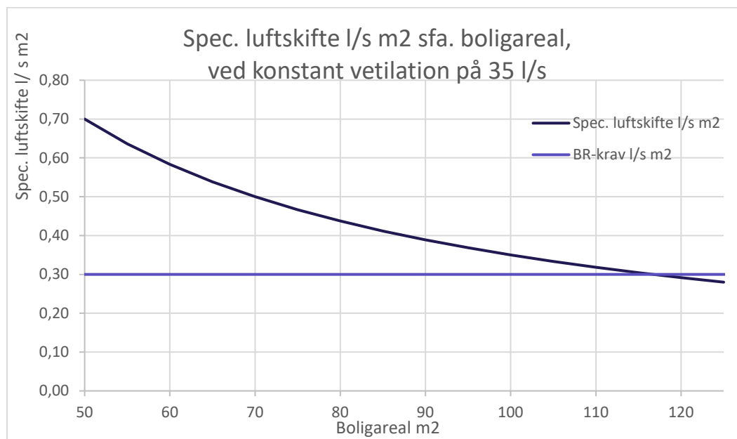
Figur 1. Luftstrømmen per boligareal ved konstant udsuget luftstrøm på 15 l/s fra bad og WC-rum og 20 l/s fra køkken for forskellige boligstørrelser. Det andet krav i BR på 0,3 l/s m² er vist som reference.
