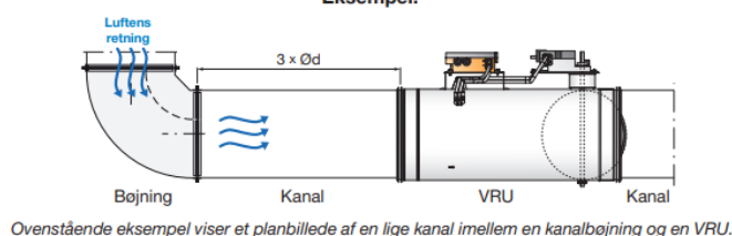
Figur 5. Fabrikat eksempel af målenøjagtighed ved volumenstrømsmåling med almindeligt målekorset. Tegning: Lindab.
