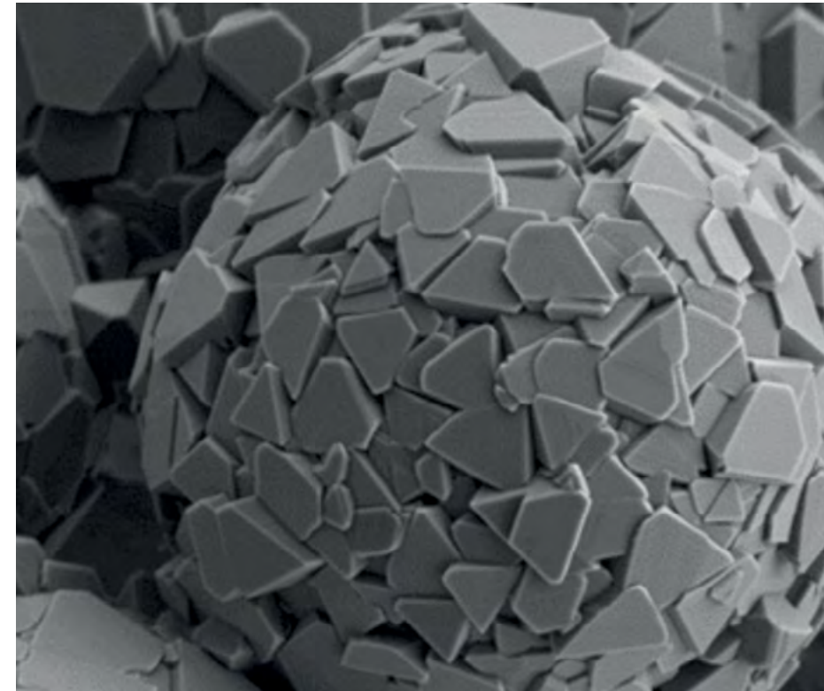
Figur 11: Visualisering af LMNO-partikler vha. scanningselektron-mikroskopi. De tætte runde partikler er udviklet for at kunne opnå høj energitæthed i LMNO-batterierne.
