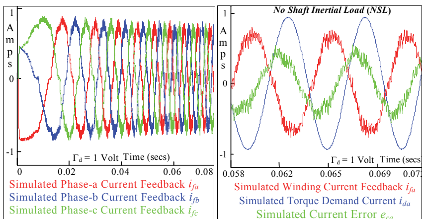
Fig. 35. BLMD 3 \Phi FC simulation I_{fj}
