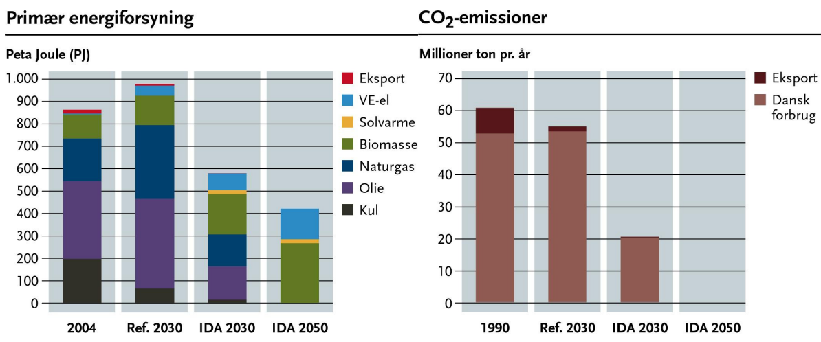
Figur 2.1: Primær energiforsyning og CO 2 -emission. CO 2 -emissionen er opdelt på den del af den danske CO 2 -emission, der kan henføres til det danske energiforbrug, og den del, der kan henføres til nettoeksporten af el.
