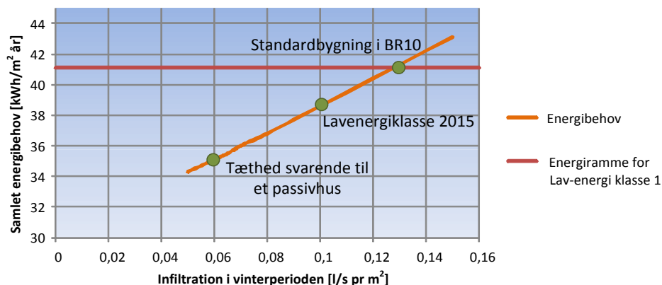
Figur 3.25. Energibehovet som funktion af infiltrationen [Larsen et al, 2011]
