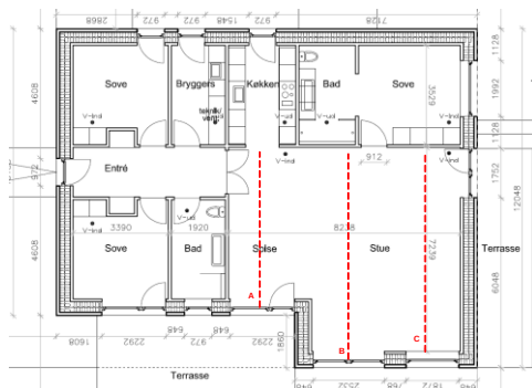
Figur 5.4: Placering af målepunkter i hus 28.
