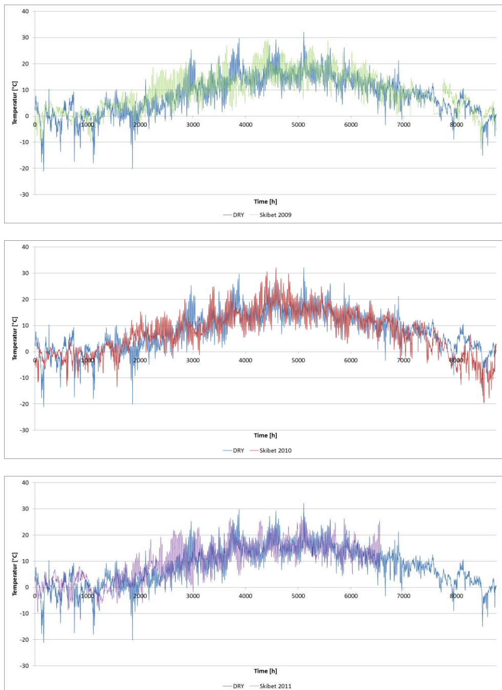
Figur E.1: Sammenligning mellem DRY og vejrdata fra skibet i hhv 2009, 2010, 2011.
