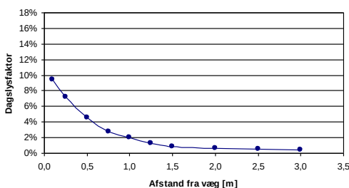
Figur 5.15: Måling af dagslysfaktor i nordvendt værelse, punkt B, hus 43.
