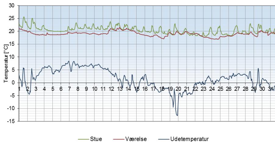
Figur 3.21. Temperaturer målt december 2009.
