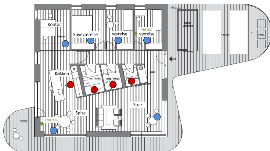
Figur 3.20. Placering af termaturmåligerne i stue og værelse (markeret med grønnt) samt indblæsning (blå cirkler) og udsugning (røde cirkler) af ventilationsluft.
