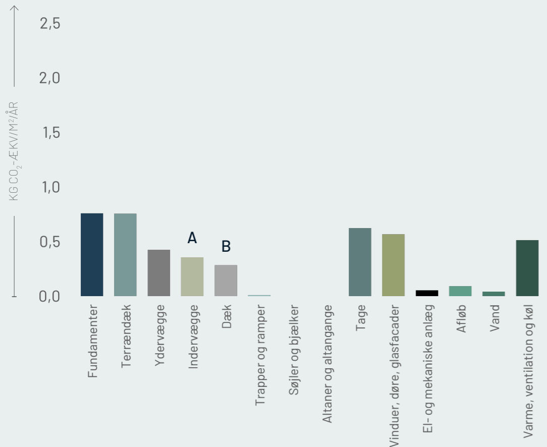
Figur R02.7: CO 2 -regnskab over byggeriets bygningsdele Den horisontale akse viser bygningens mest centrale bygningsdele, herunder fundamenter, terrændæk, ydervægge, indervægge, dæk, trapper og ramper, søjler og bjælker, altaner og altangange, tage, vinduer, døre og glasfacader, el- og mekaniske anlæg samt tekniske installationer (standard værdier).
