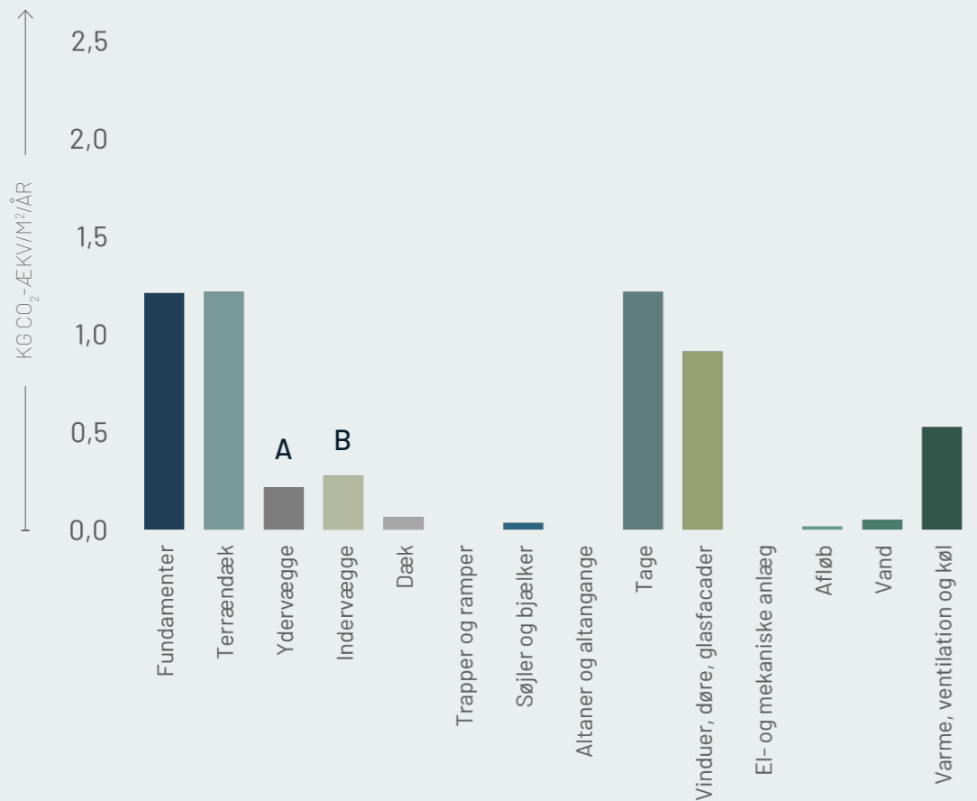
Figur ENF09.7: CO 2 -regnskab over byggeriets bygningsdele Den horisontale akse viser bygningens mest centrale bygningsdele, herunder fundamenter, terrændæk, ydervægge, indervægge, dæk, trapper og ramper, søjler og bjælker, altaner og altangange, tage, vinduer, døre og glasfacader, el- og mekaniske anlæg samt tekniske installationer (standard værdier).
