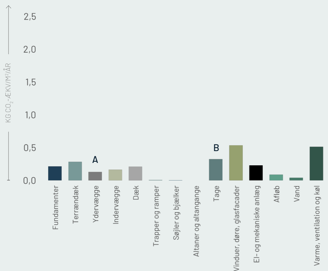
Figur R01.7: CO 2 -regnskab over byggeriets bygningsdele
