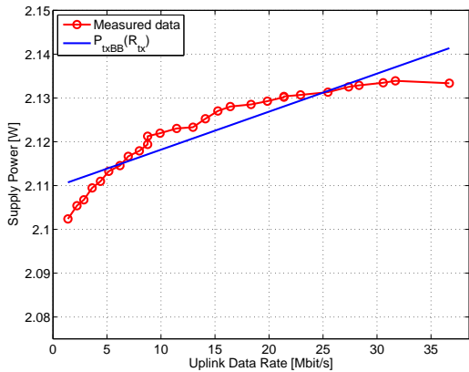
Fig. 5. Transmit BB.
