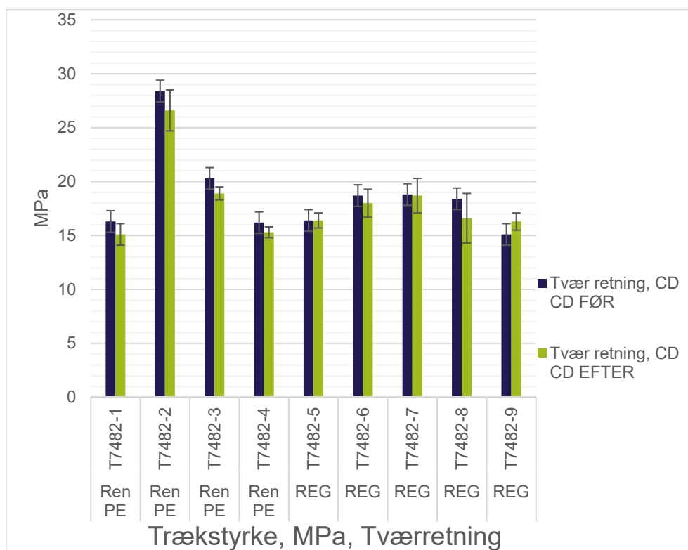
FIGUR 37. Trækstyrke af PE-membraner, før og efter accelereret ældning for længderetningen (MD, Machine Direction). 'Ren PE' er PE-membraner af ren PE. 'REG' er PE-membraner af eller indeholdende regenereret PE.
