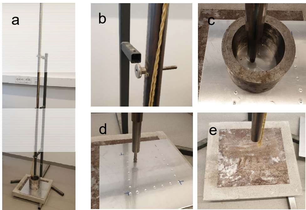
FIGUR 16. Opstilling til måling af slagpåvirkning. (a) hele opstillingen, (b) split til indstilling af faldhøjde, (c) stålcyllinder og aluminiumsplade, hvorimellem membranstykket holdes fast, (d) aluminiumsplade med mærker efter målinger, og (e) ballast-flise af beton med indstøbt stålplade.
