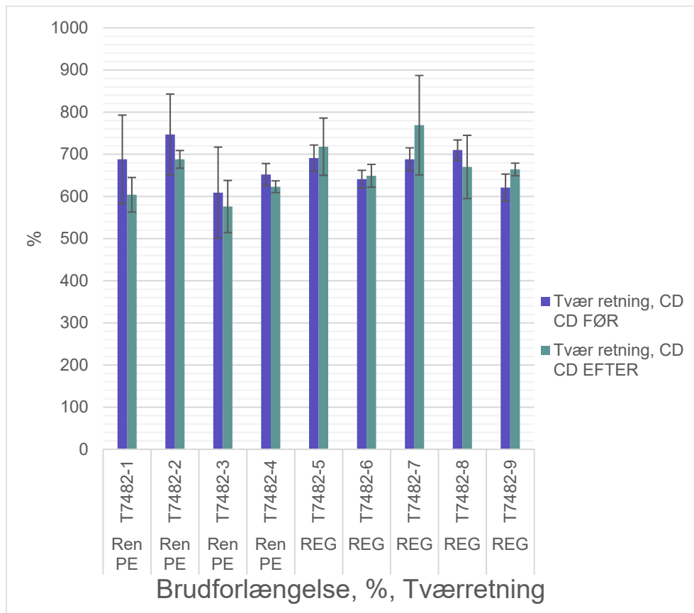
FIGUR 39. Brudforlængelsen af PE-membraner, før og efter accelereret ældning for tværreretningen (CD, Cross Direction). 'Ren PE' er PE-membraner af ren PE. 'REG' er PE-membraner af eller indeholdende regenereret PE.
