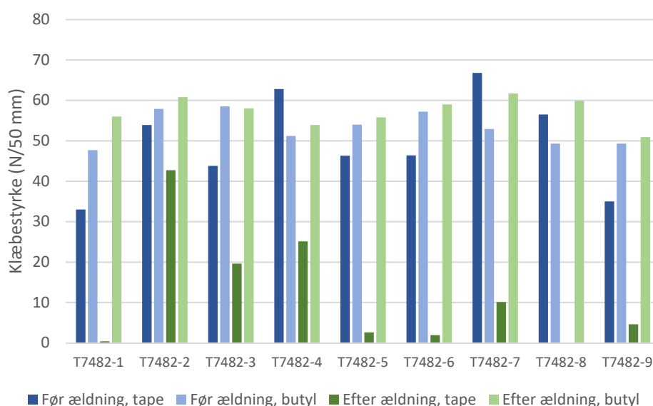
FIGUR 56. Peel klæbestyrke (middelværdier af 7 målinger) for PE-membransystemer før og efter accelereret ældning for tapet samling (tape) og til sammenligning klæbestyrke mellem membraner samlet med bånd af butyl.
