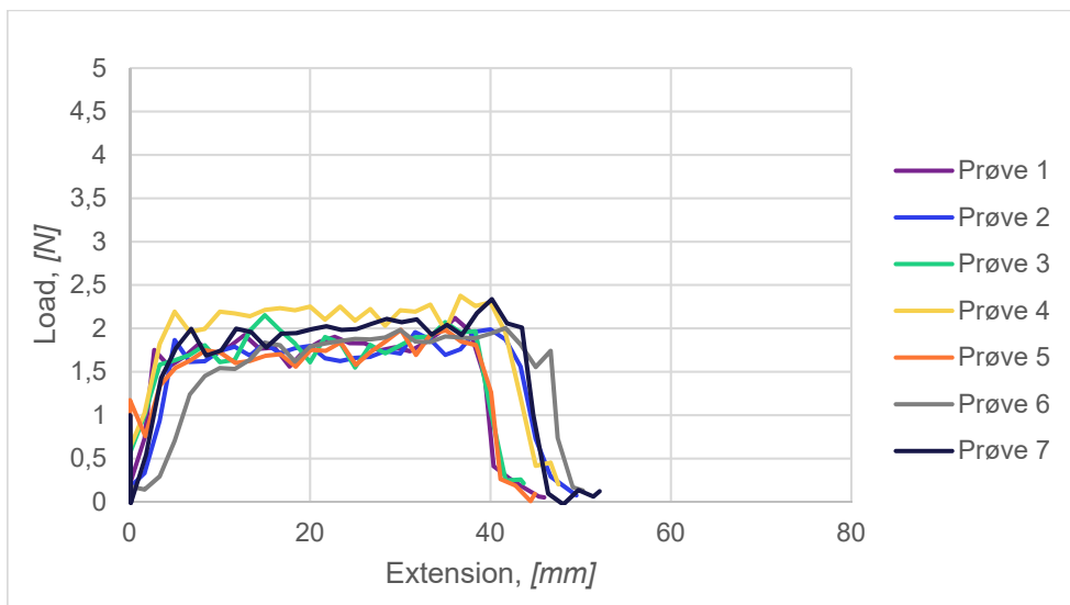
FIGUR 49. Peel klæbestyrke for tapet samling efter accelereret ældning, måling af gennemsnittlig peelstyrke for PE-membran T7482-6.
