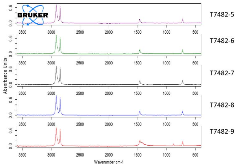
FIGUR 25. ATR-FTIR spektre af membraner som indeholder regenereret PE viser, at alle membranerne er baseret på lavdensitetspolyethylen med uorganiske tilsætningsstoffer.
