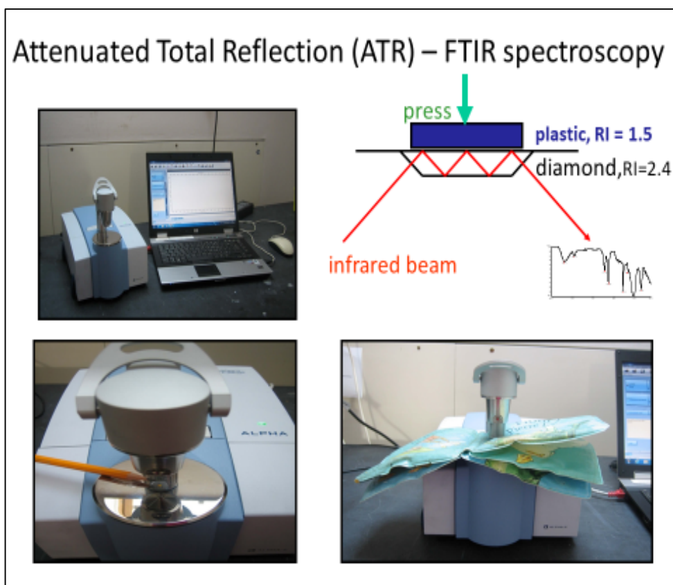
FIGUR 6. ATR-FTIR spektroskopi blev brugt til at analysere membranerne på Nationalmuseet.
