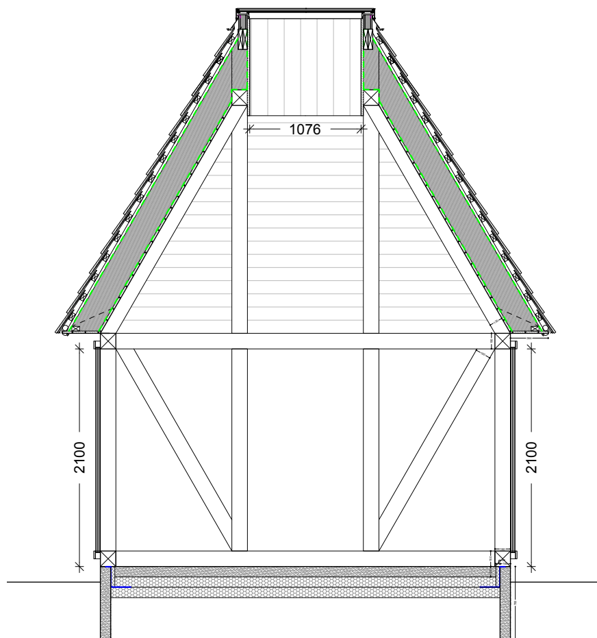
KORT SNIT 1:50
